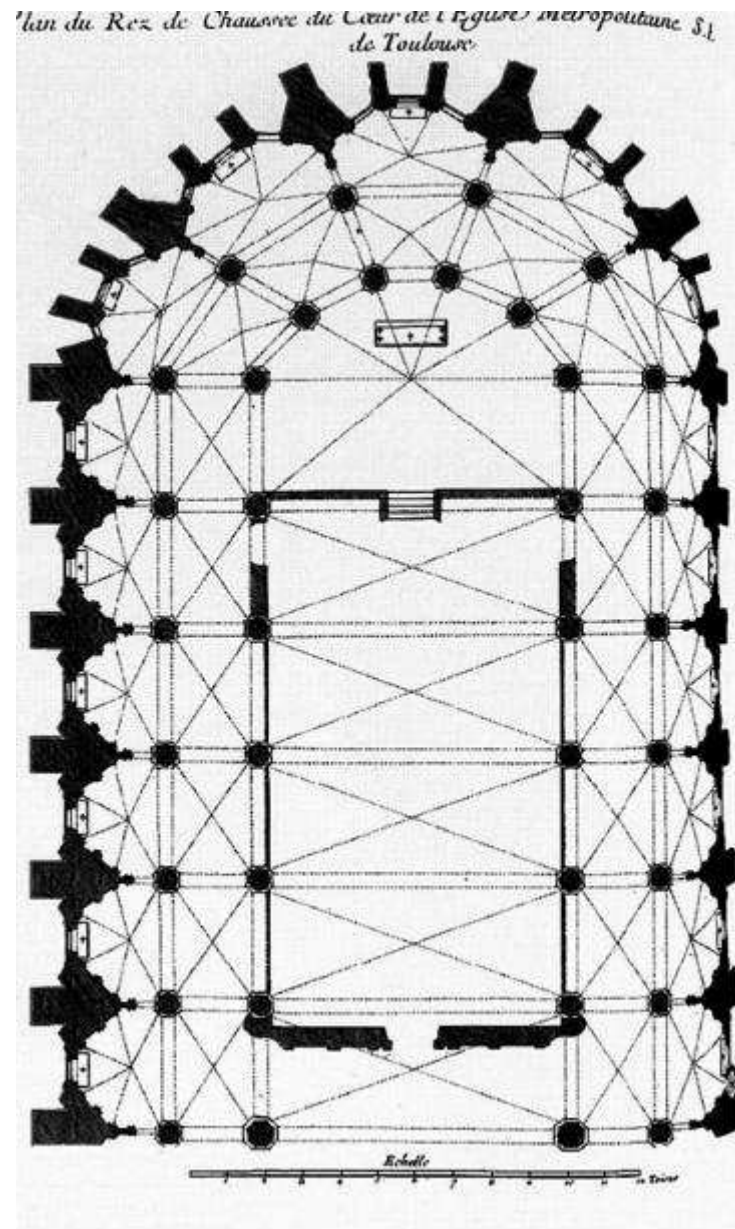
TOULOUSE, KATEDRALA ST-ETIENNE, půdorys, lod' první polovina a třetí čtvrtina 13. stol., počátek stavby chóru po 1270.
